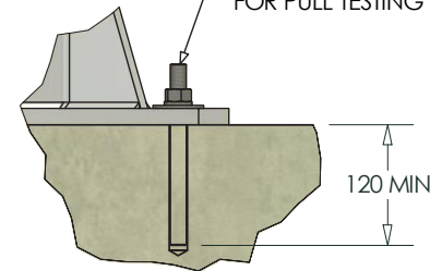
DETAIL Z ( 1 : 8 )
