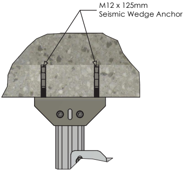
DETAIL X ( 1 : 10 )
