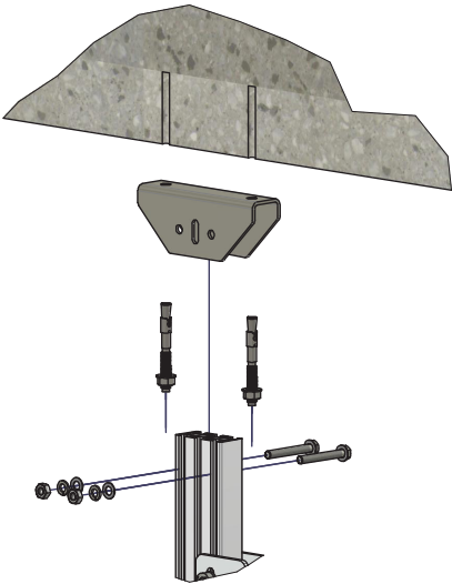
DETAIL Y ( 1 : 10 )
